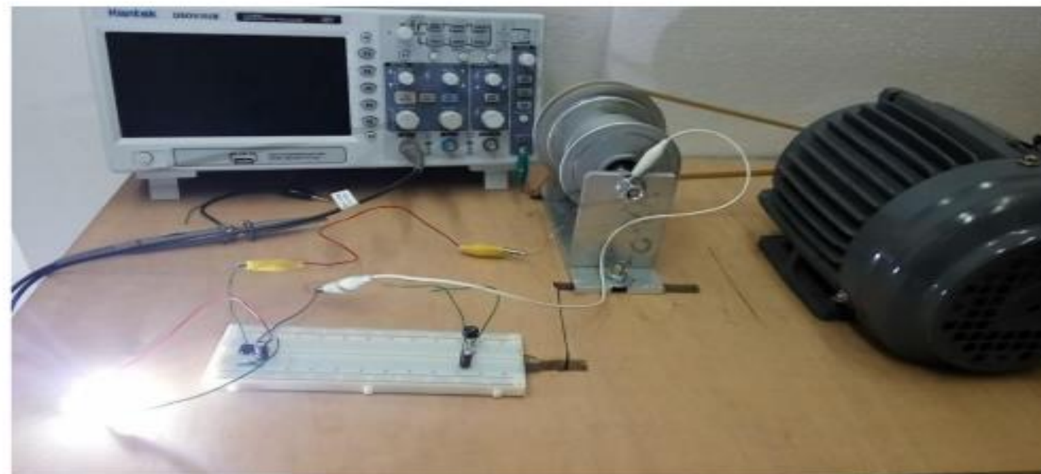
使用改良後的發電花鼓，產生3V 電壓，讓3V1W LED 燈發亮
